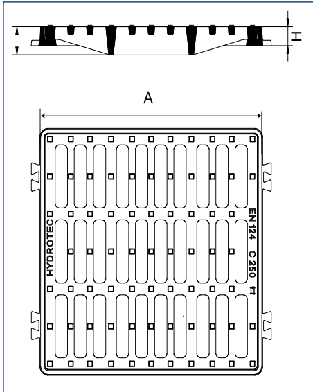
▲ Art. Nr. 323 Einlaufgitter quadratisch aus Sphäroguss
